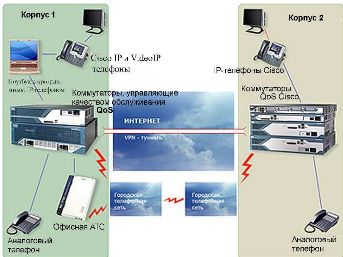
Рис. 4.2.1 - Схема работы IP-телефонии
