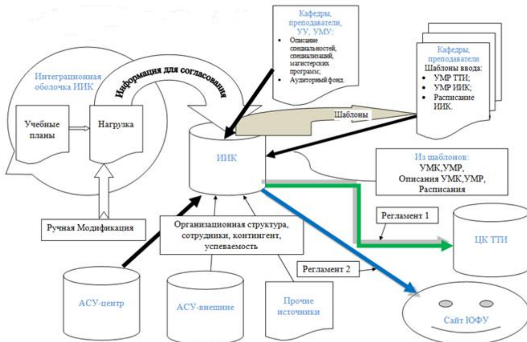
Рис. 4.1.1 - Общая схема информационных потоков
